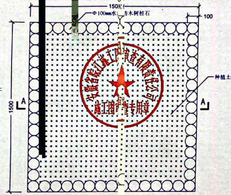
弋江北路树池平面图 (水泥仿木树桩)
